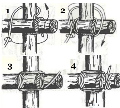
Vinkelbesnøring.
