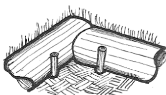
DETAIL AF KANTBESKYTTELSE FOR BÅLPLADS
